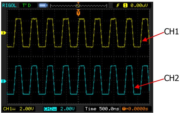
图 2-4 恢复延时后
