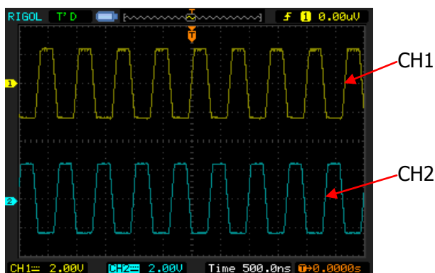
图 2-3 恢复延时前
