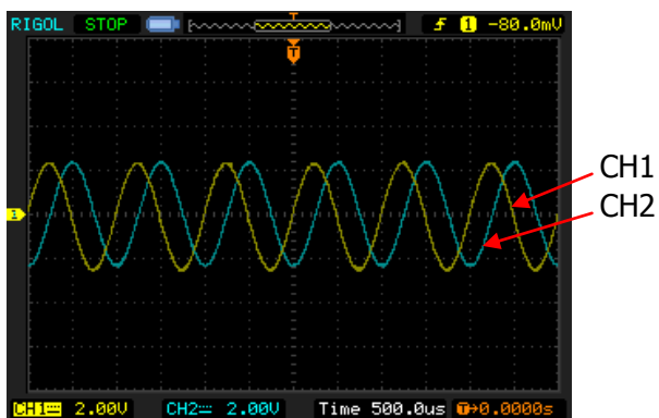
图 2-1 同相位前
