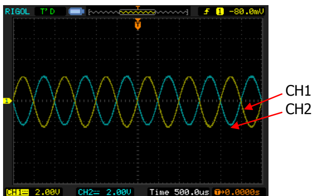
图 2-2 同相位后
