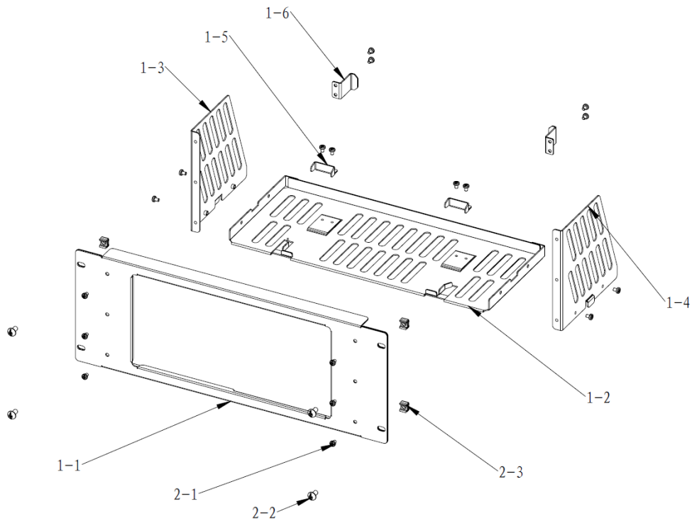
图 1-11 机架部件
