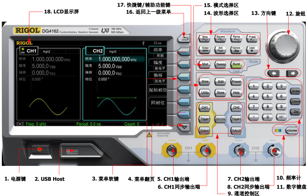
图 1-5 DG4000 前面板
