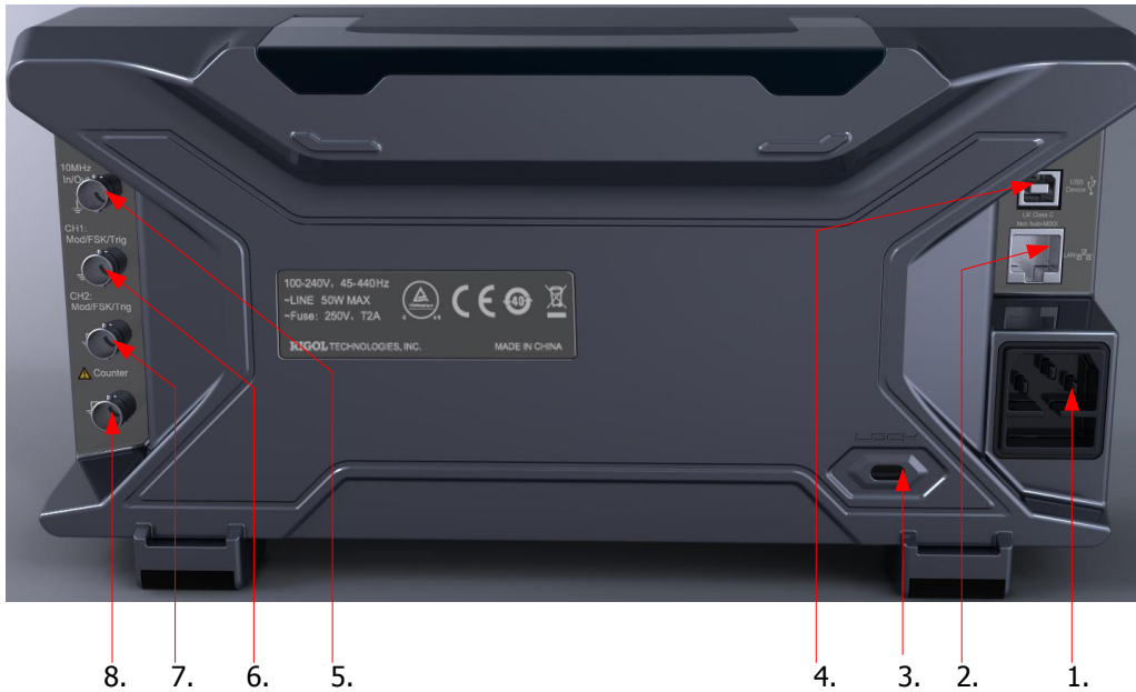
图 1-6 DG4000 后面板
