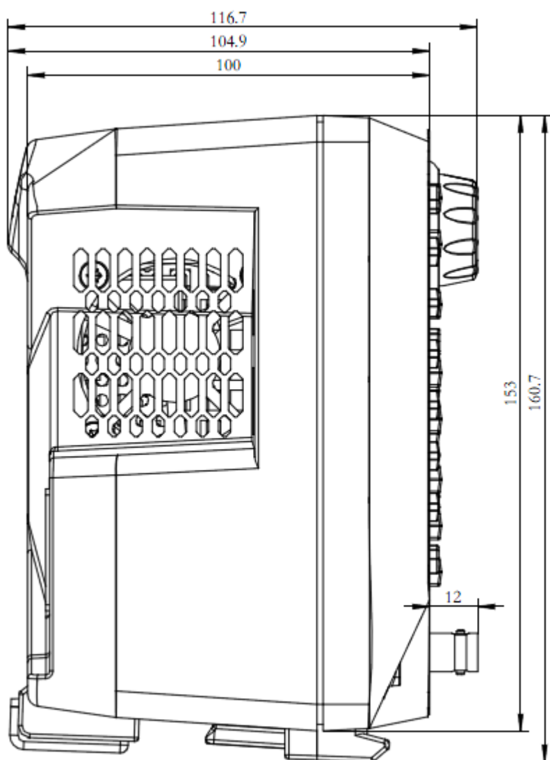
图 1-4 侧视图
